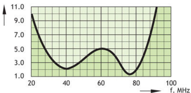
Typischer SWR Verlauf
