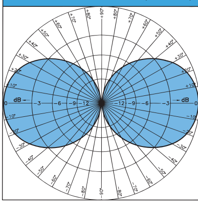
TYP. STRAHLUNGSDIAGRAMM (VERTIKAL)
