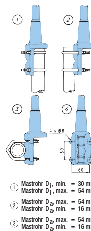
UNIVERSAL-MONTAGEBESCHLAG:
