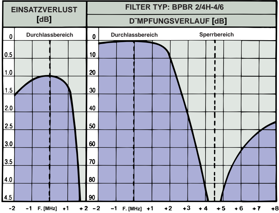
TYPISCHER KURVENVERLAUF @ 4.5 MHz DUPLEXABSTAND:
