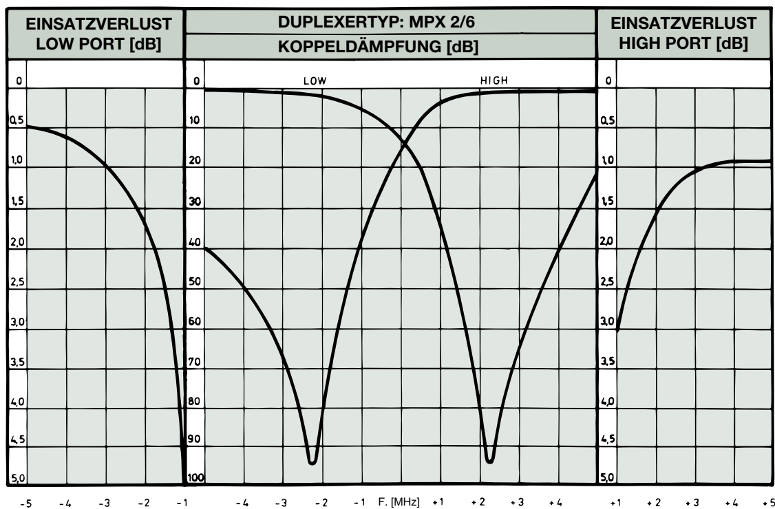
TYPISCHER KURVENVERLAUF @ 5 MHz DUPLEXABSTAND:
