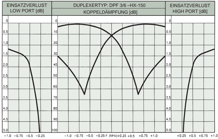
TYPISCHER KURVENVERLAUF @ 1.3 MHz DUPLEXABSTAND:
