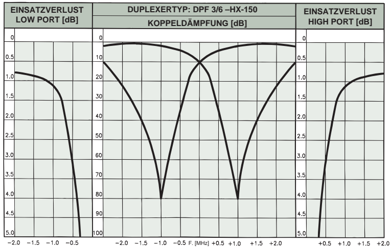
TYPISCHER KURVENVERLAUF @ 2 MHz DUPLEXABSTAND:
