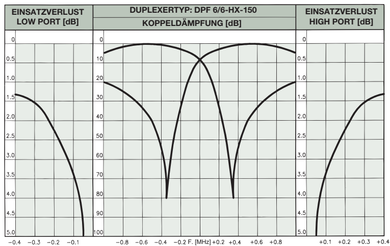
TYPISCHER KURVENVERLAUF @ 0.7 MHz DUPLEXABSTAND:
