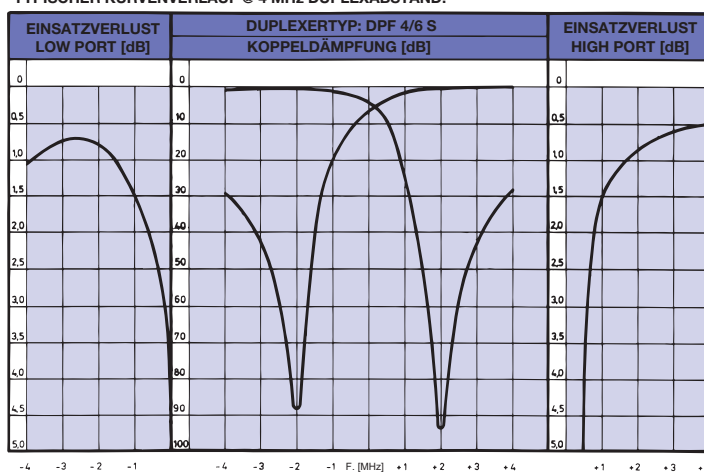
TYPISCHER KURVENVERLAUF @ 4 MHz DUPLEXABSTAND:
