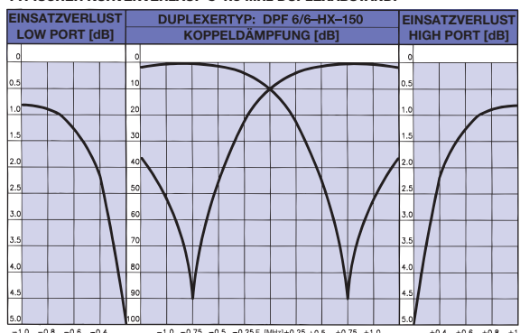
TYPISCHER KURVENVERLAUF @ 1.5 MHz DUPLEXABSTAND:
