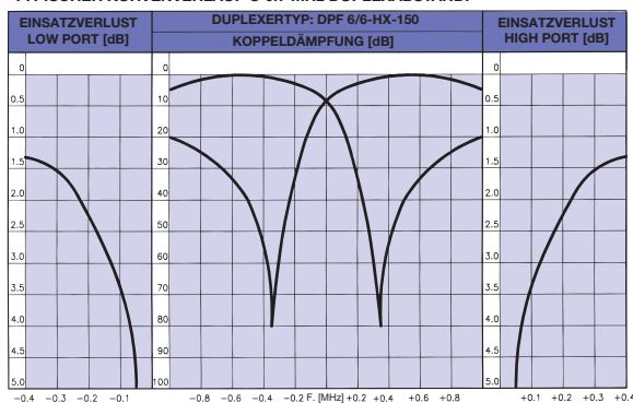
TYPISCHER KURVENVERLAUF @ 1.5 MHz DUPLEXABSTAND:
