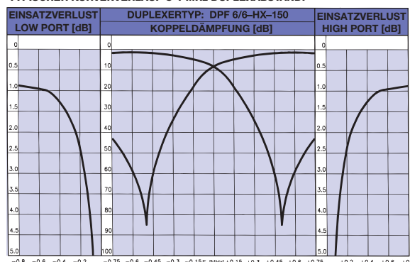
TYPISCHER KURVENVERLAUF @ 1 MHz DUPLEXABSTAND:
