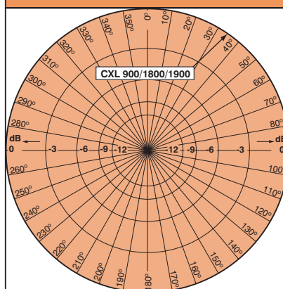
TYP. STRAHLUNGSDIAGRAMM (HORIZONTAL)
