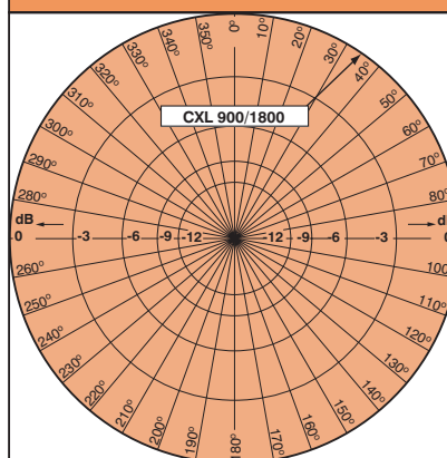
TYP. STRALUNGSDIAGRAMM (HORIZONTAL)
