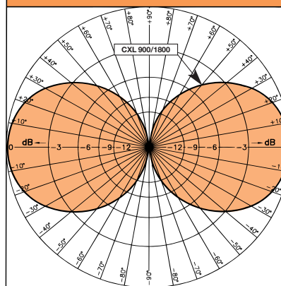
TYP. STRALUNGSDIAGRAMM (VERTIKAL)
