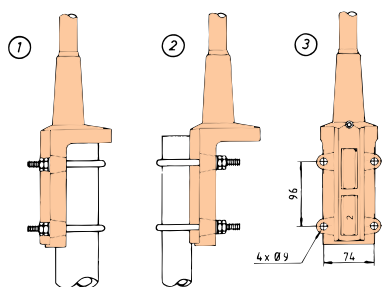
UNIVERSAL-MONTAGEBESCHLAG
