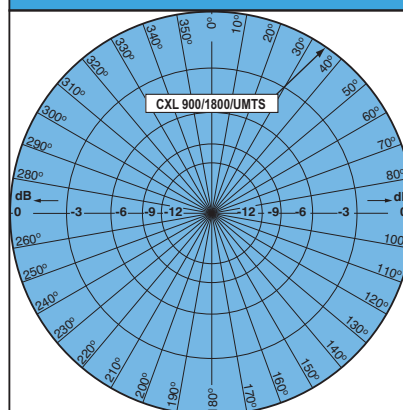
PATRÓN TÍPICO DE RADIACIÓN (PLANO H)
