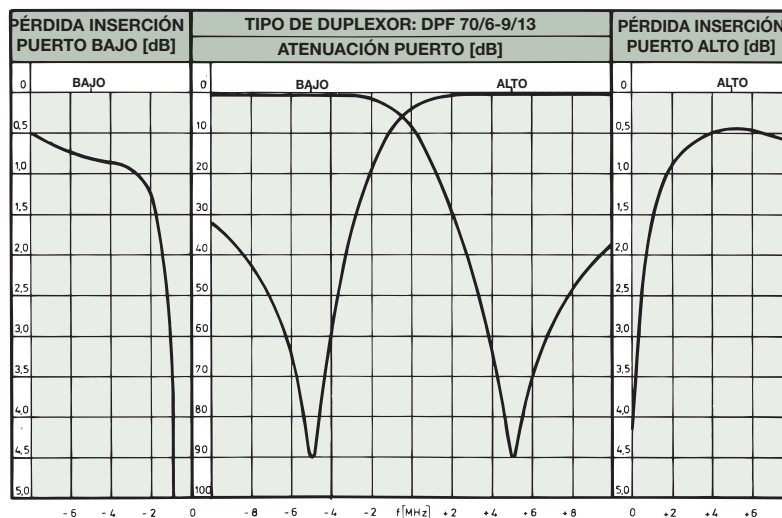
CURVAS TÍPICAS DE RESPUESTA @ ESPACIADO DE 10 MHz:
