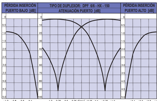
CURVAS TÍPICAS DE RESPUESTA @ ESPACIADO DUPLEX DE 1.5 MHz:
