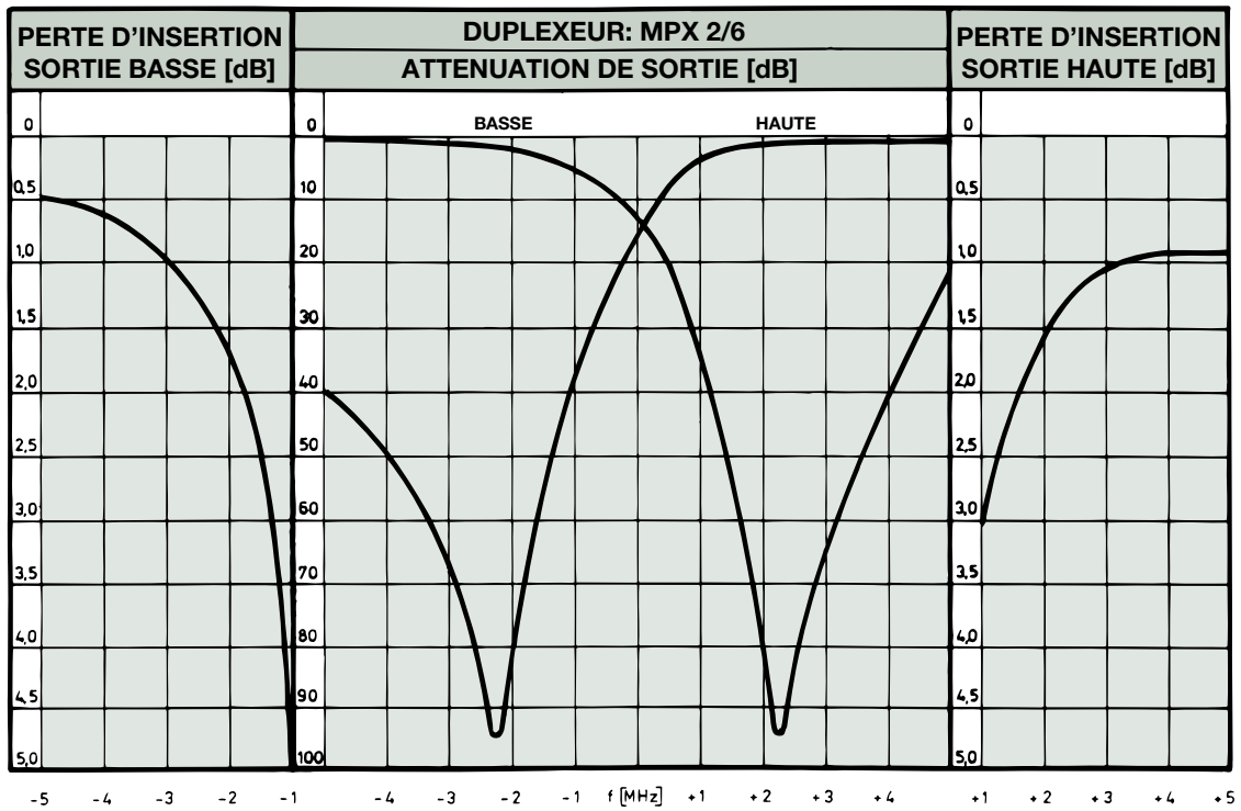
COURBES DE REPONSE TYPIQUES ECART DUPLEX à 5 MHz:
