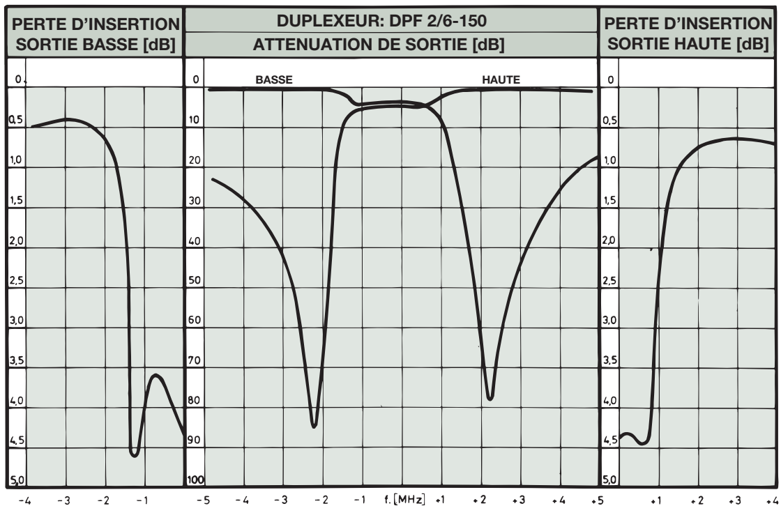
COURBES DE REPONSE TYPQUES ECART DUPLEX à 4,5 MHz:
