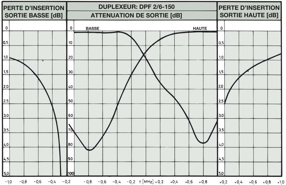
COURBES DE REPONSE TYPQUES ECART DUPLEX à 1,6 MHz:
