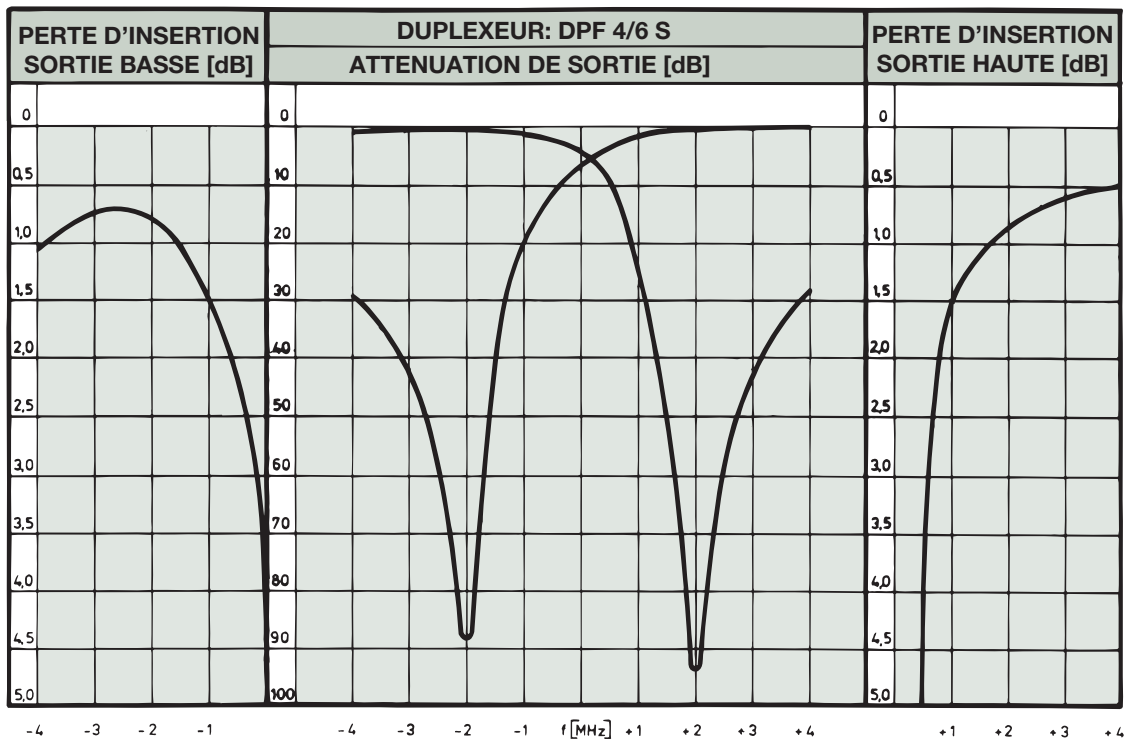
COURBES DE REPONSE TYPIQUES ECART DUPLEX à 4 MHz:
