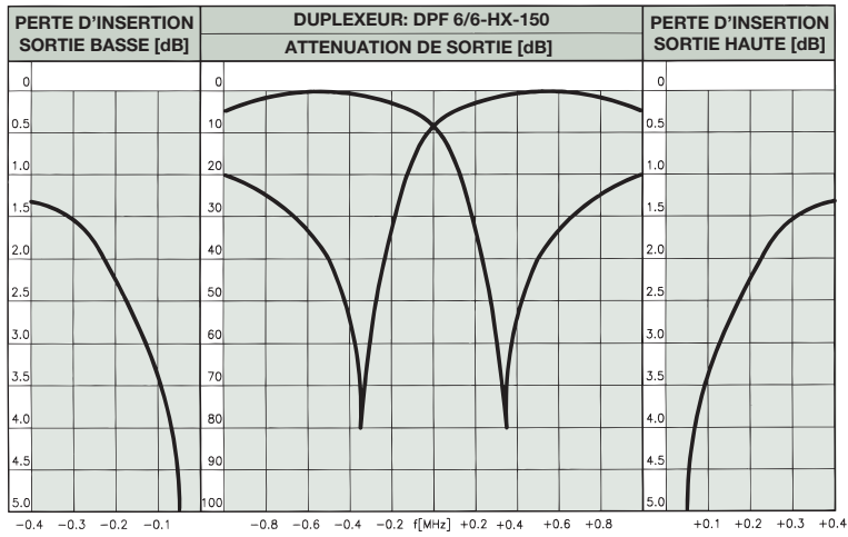
COURBES DE REPONSE TYPIQUES ECART DUPLEX à 0,7 MHz:
