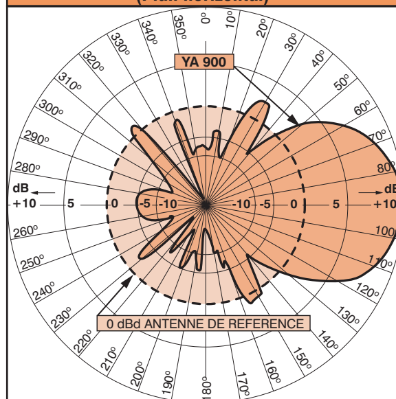
DIAGRAMME DE RAYONNEMENT TYPIQUE (Plan horizontal)
