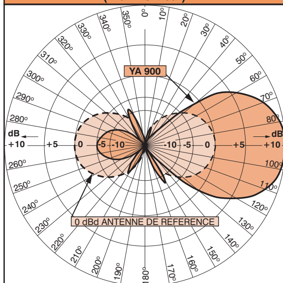
DIAGRAMME DE RAYONNEMENT TYPIQUE (Plan vertical)
